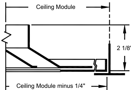
Border Type 3 (Lay-In)
